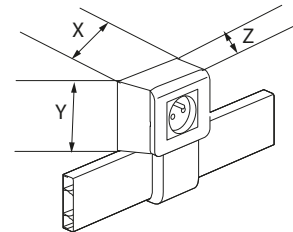
Cotes d'encombrement
