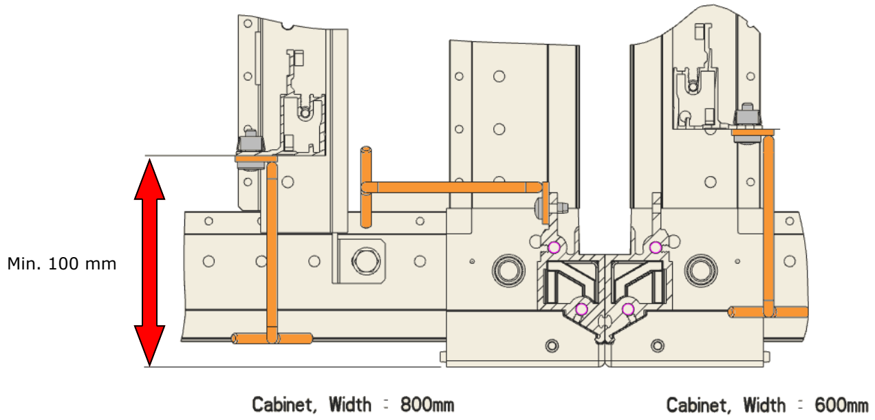
Vue de dessus — Top
