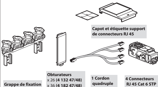
Grappe de fixation
