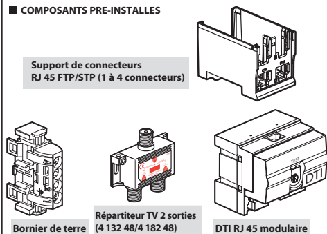
Bornier de terre
