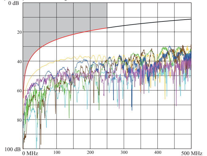
ELFEXT (Equal Level End Crosstalk Attenuation) (Atténuation télé diaphonique de niveau égal)
