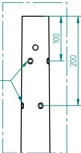
DETAIL B TETE DE MAT AVEC OPTION CREVES POLE HEAD WITH THREADED HOLES
