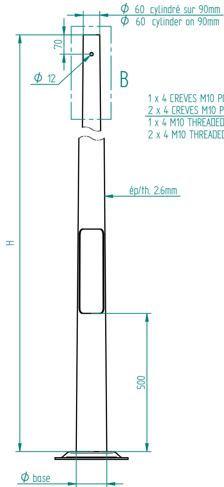
DETAIL B TETE DE MAT AVEC OPTION CREVES POLE HEAD WITH THREADED HOLES
