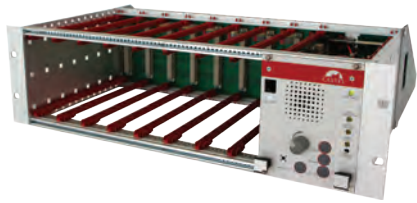
CASI Centrale d'alarme et de sécurité interphonique REF 220.5000
