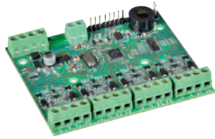
EP708 Extension filaire sur bus REF 320.2185
