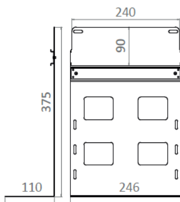
Dimension – plan coupe
