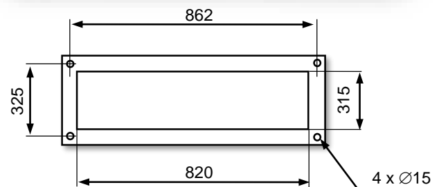
Schéma d'implantation au sol
