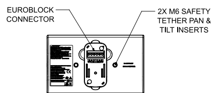
Vue arrière
