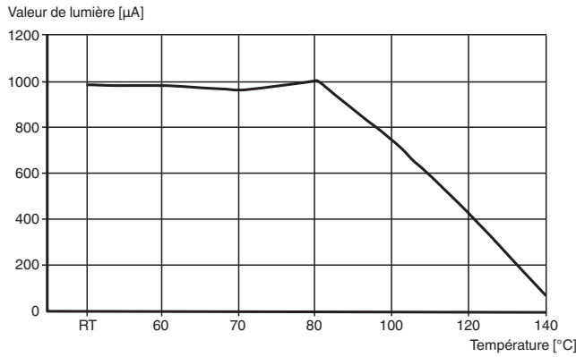
Relation entre la valeur de réflectance et la température (mesurée à chaud)
