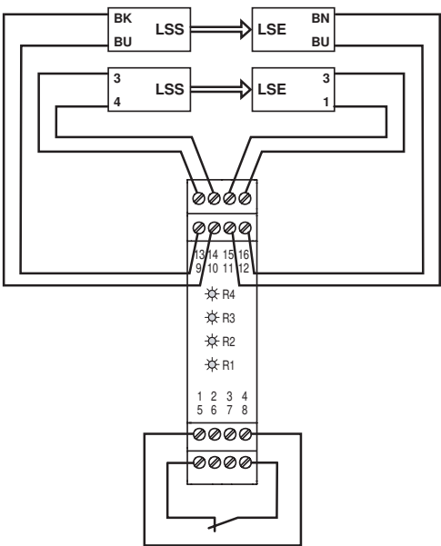
Exemple de raccordement (LSS = émetteur cellule photoélectrique ; LSE = récepteur cellule photoélectrique)
