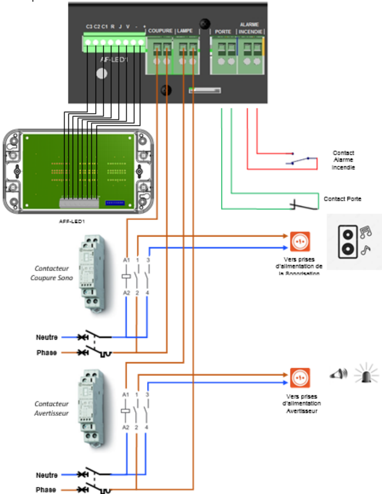
Fig. VII : Raccordements des contacts
