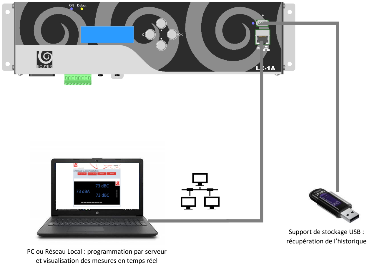
Fig. VIII : Raccordements Face Avant
