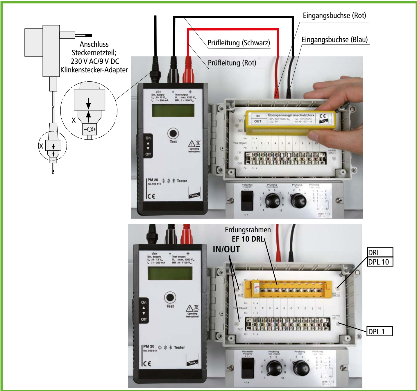
Figur 4 Prüfaufbau 2
