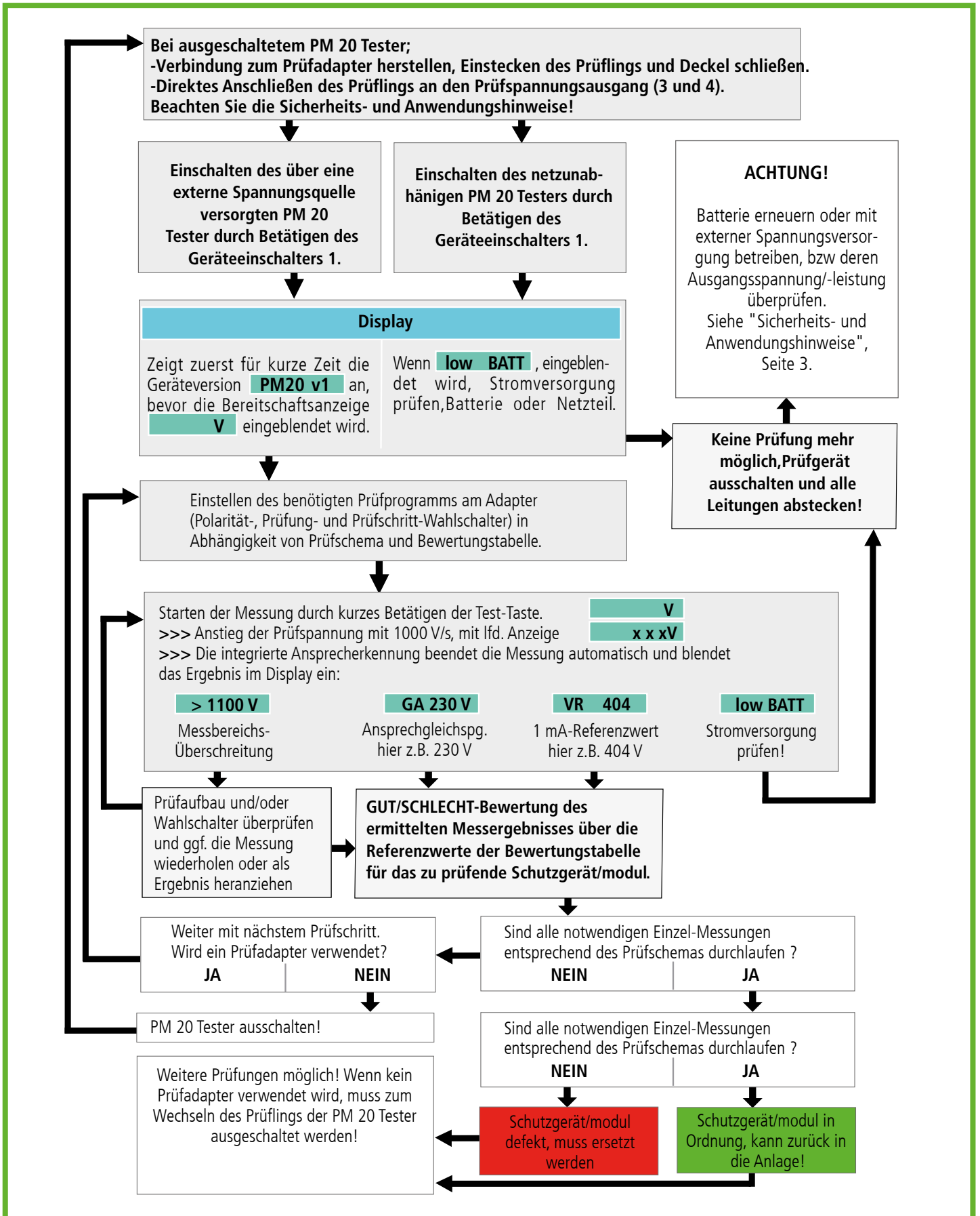
Figur 6 Prüfablauf
