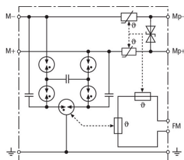
Schéma de principe du circuit BVT KKS APD 36
