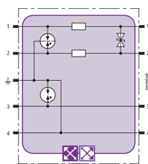
Schéma de principe du circuit BXT ML2 BD DL S 15
