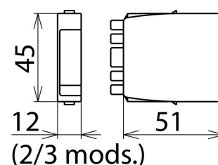
Dimensions BXT ML4 B 180
