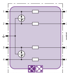
Schéma de principe du circuit BXT ML4 B 180
