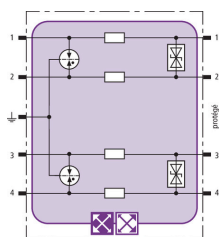
Schéma de principe du circuit BXT ML4 BD HF 5
