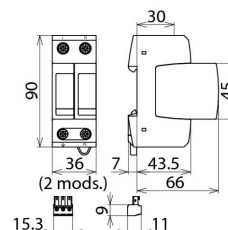
Dimensions DG M TT 2P 275 FM
