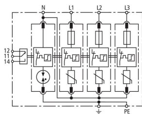
Schéma de principe du circuit DG M TT 5 CI 275 NL FM
