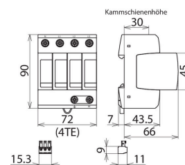
Dimensions DG M TNS 275 NL FM
