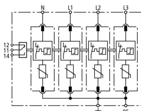
Schéma de principe du circuit DG M TNS 275 NL FM
