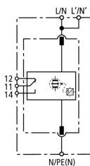
Schéma de principe du circuit DB M 1 150 FM
