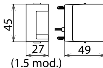
Dimensions DG MOD E DC 550
