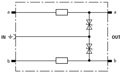
Schéma de principe du circuit DRL RE 60
