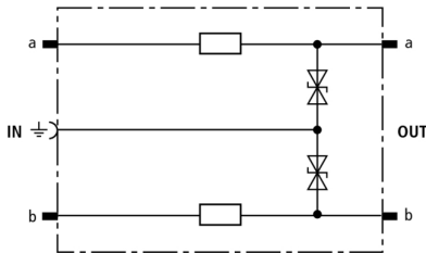
Schéma de principe du circuit DRL RE 180
