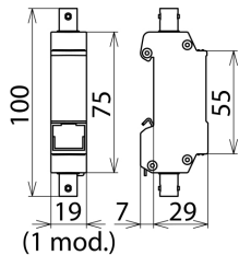
Dimensions DGA BNC VCD
