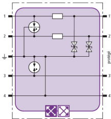
Schéma de principe du circuit BXT ML2 BE S 48
