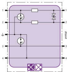
Schéma de principe du circuit BXT ML2 BD S 24
