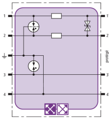
Schéma de principe du circuit BXT ML2 BD S 48
