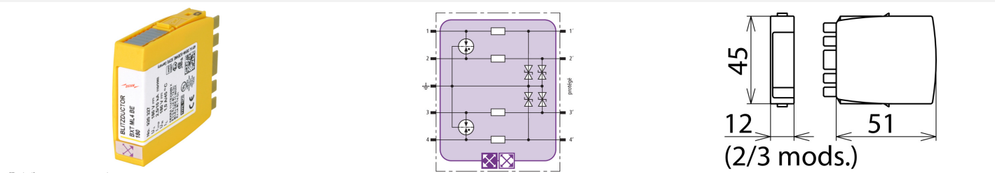
Illustrations sans engagement Schéma de principe du circuit BXT ML4 BE 180 Dimensions BXT ML4 BE 180
