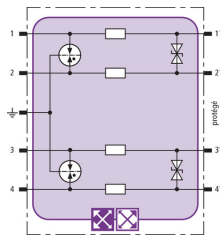
Schéma de principe du circuit BXT ML4 BD 24
