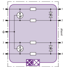
Schéma de principe du circuit BXT ML4 BD 48
