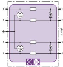
Schéma de principe du circuit BXT ML4 BD 60
