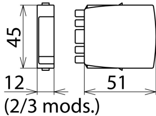
Dimensions BXT ML4 BD 60
