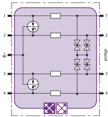
Schéma de principe du circuit BXT ML4 BC 5
