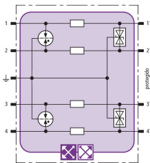
Schéma de principe du circuit BXT ML4 BE HF 5
