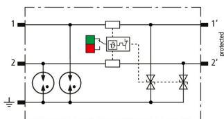
Circuit du BCO ML2 BE 48
