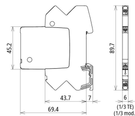
Dimension du BCO ML2 BE 48
