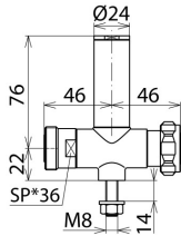
Dimensions DGA L4 7 16 S
