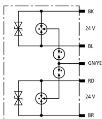
Schéma de principe du circuit DPI CD EXI+D 2X24 N
