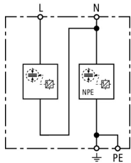
Schéma de principe du circuit DSH TT 2P 255
