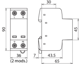
Dimensions DSH TT 2P 255
