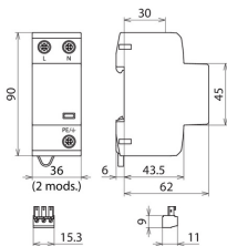
Dimensions DSH TN 255 FM
