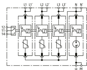
Schéma de principe du circuit DG MP TT 275 FM
