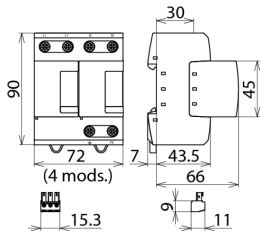
Dimensions DV M TT 2P 255 FM
