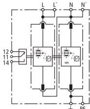
Schéma de principe du circuit DV M TT 2P 255 FM
