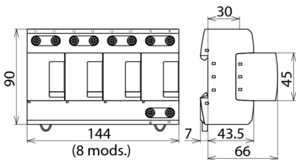
Dimensions DV M TNS 255
