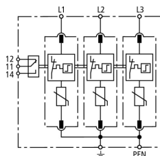
Schéma de principe du circuit DG M TNC 275 FM
