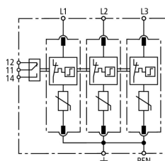
Schéma de principe du circuit DG M TNC 440 FM
