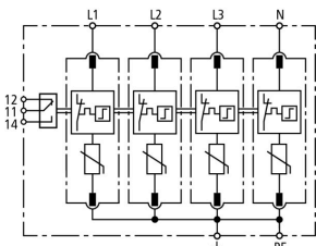
Schéma de principe du circuit DG M TNS 275 FM
