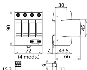
Dimensions DG M TNS 275 FM
