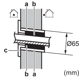
a Tuyauterie encastrée b Mastic c Couvercle du trou de mur
