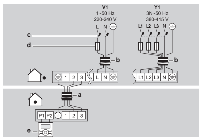
a Câble d'interconnexion b Câble d'alimentation c Disjoncteur de protection contre les fuites à la terre d Fusible e Interface utilisateur
