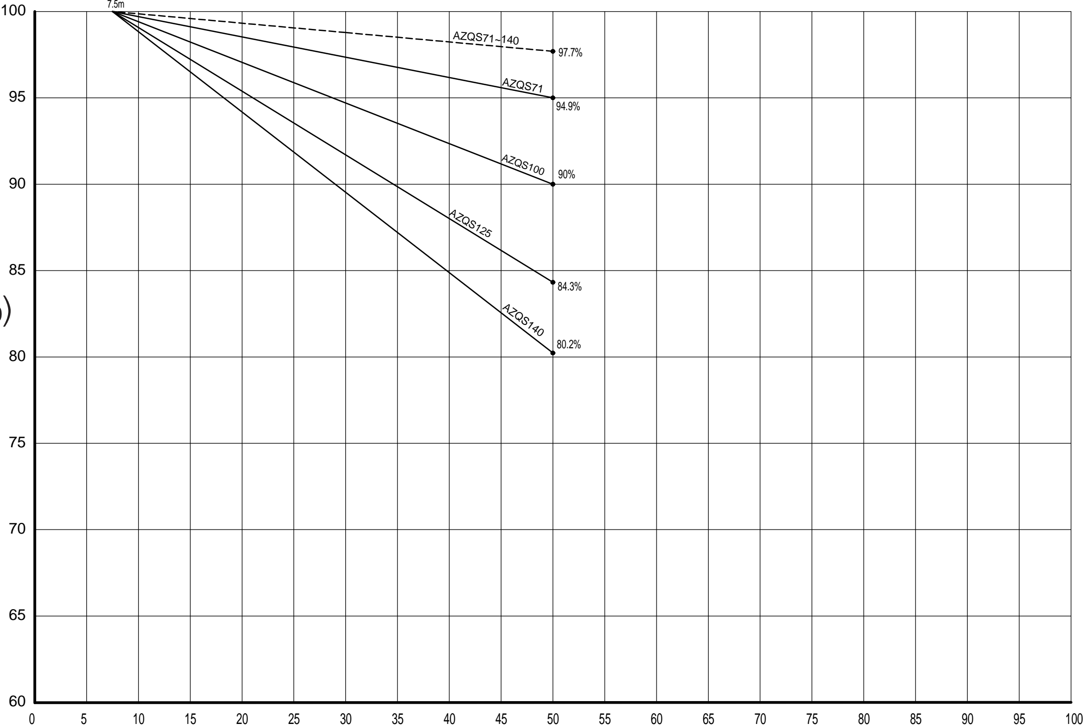
Puissance en fonction de la longueur de tuyauterie sur site pour système avec inverter
