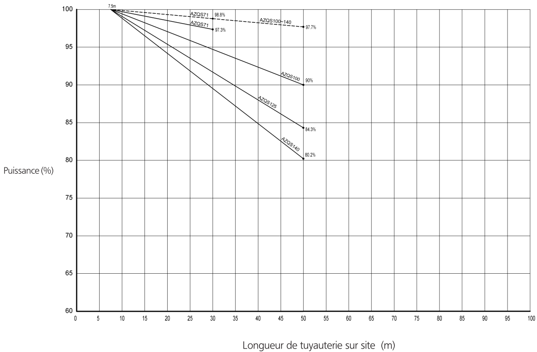
Puissance en fonction de la longueur de tuyauterie sur site pour système avec inverters
